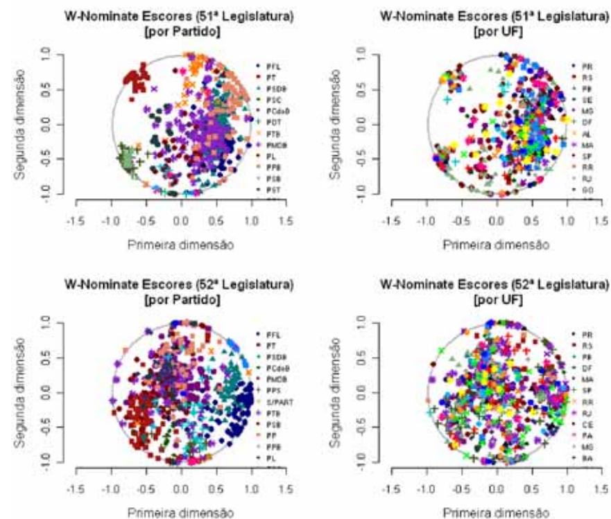
FIGURA 1. Escores do W-Nominate (51ª e 52ª legislaturas)
