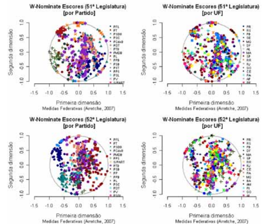
FIGURA 2. Escores do W-Nominate para Medidas Federativas (Arretche, 2007)
