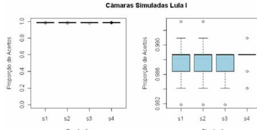
FIGURA 4. Real x Simulado (Lula I)
