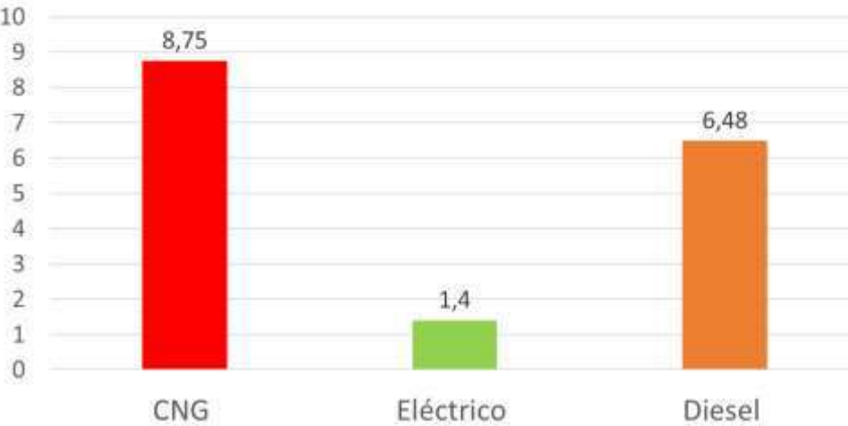
Consumo Energía (kWh/km)
