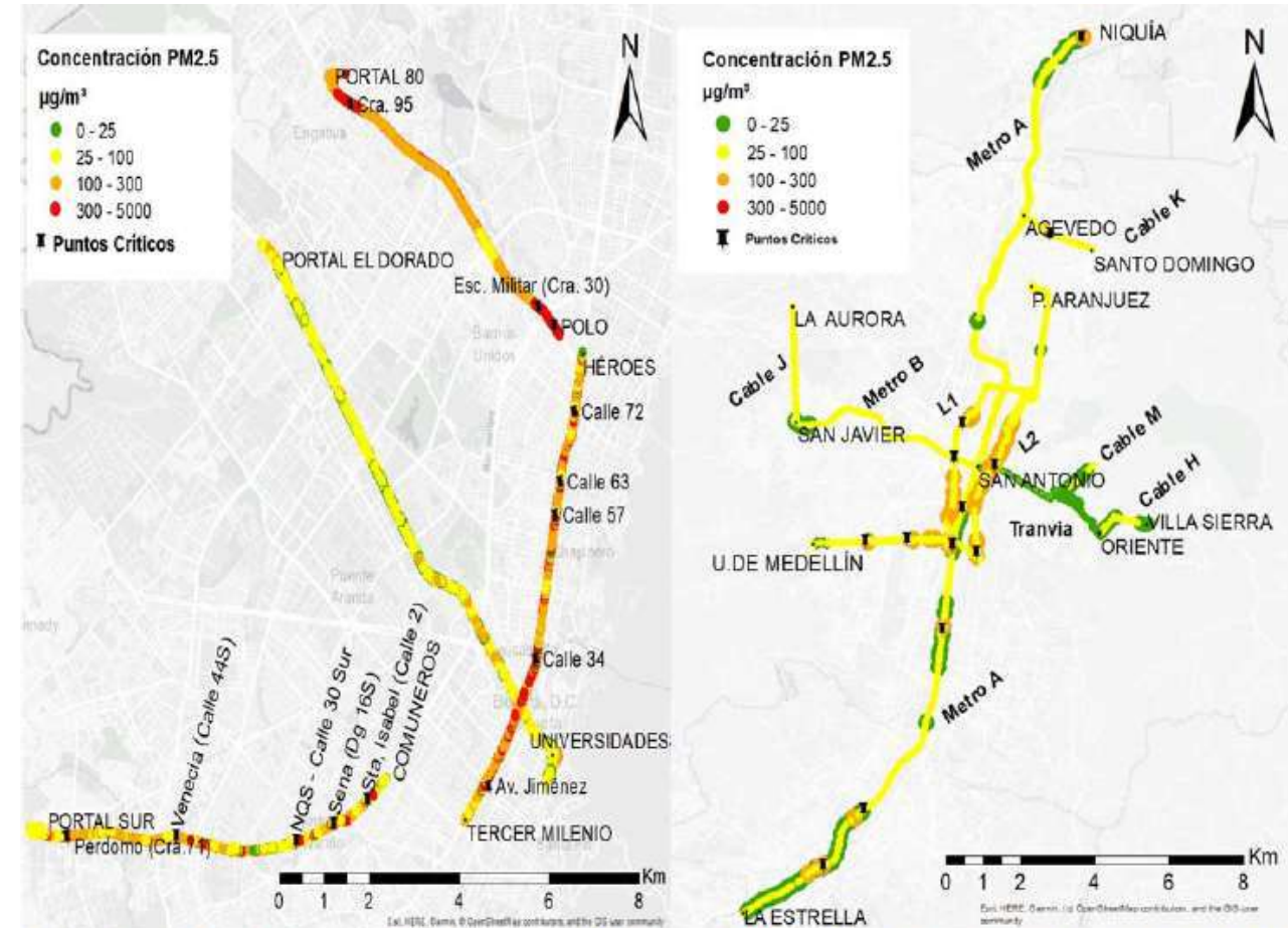
Fig. 2a. Distribución PM 2.5 TransMilenio Fig. 2b. Distribución PM 2.5 SITVA
